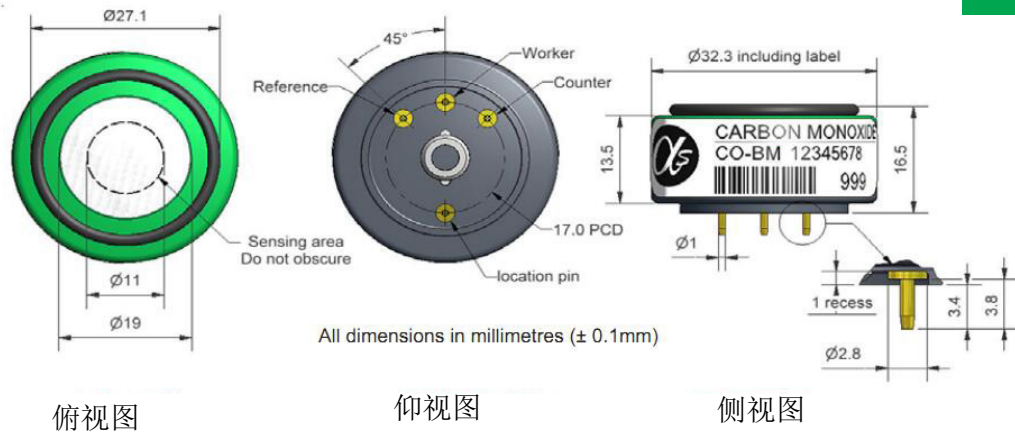
图1 CO-BM示意图
