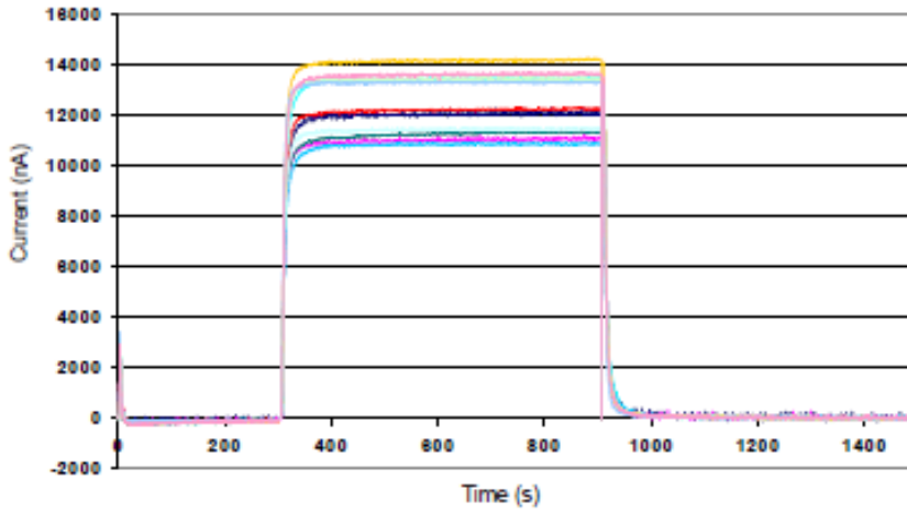
图5 H 2 S通道对25ppm H 2 S的响应
