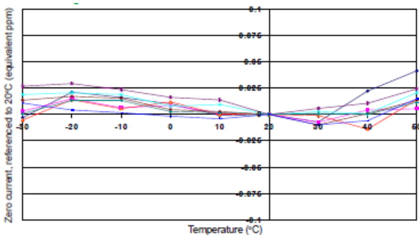
图7 H 2 S通道零点温度特性
