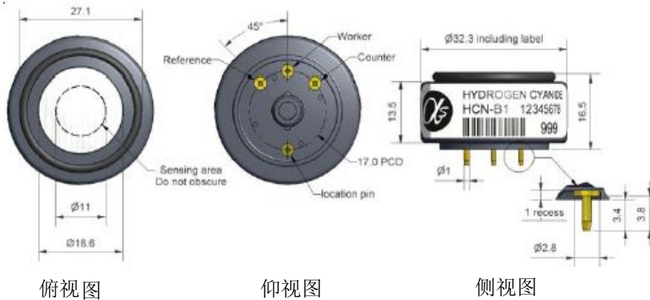
图1 HCN-B1示意图
